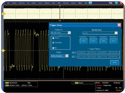
► Protocol Trigger.
