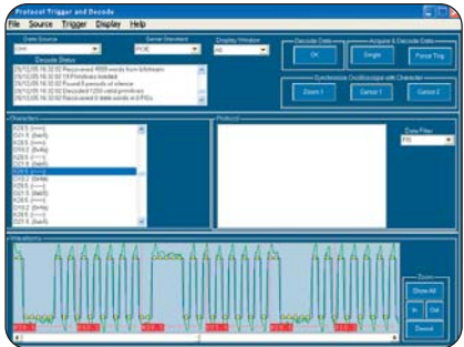
► Protocol Decode.
